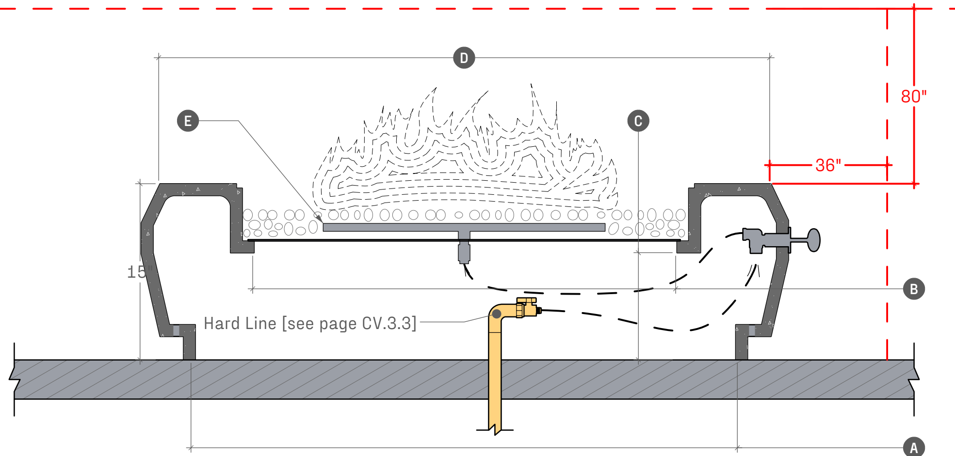
CV.2.1 SECTION DETAIL SCALE: 1" = 0' - 8"
