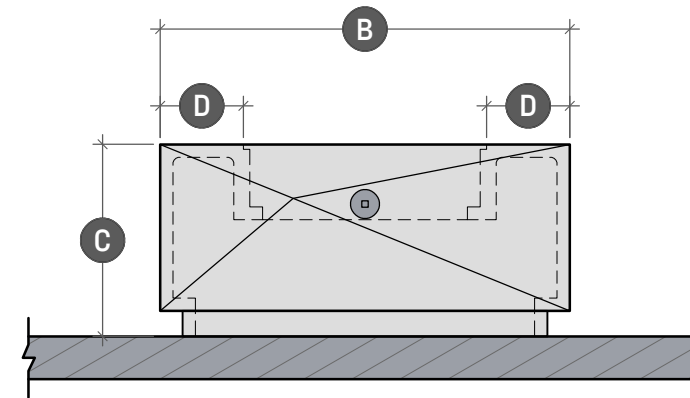
CV.1.3 SIDE ELEVATION SCALE: 1" = 1' - 3"
